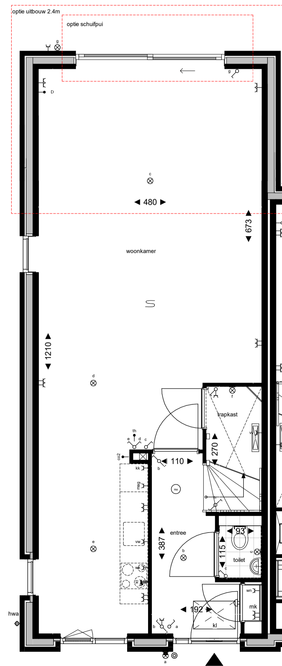
begane grond
