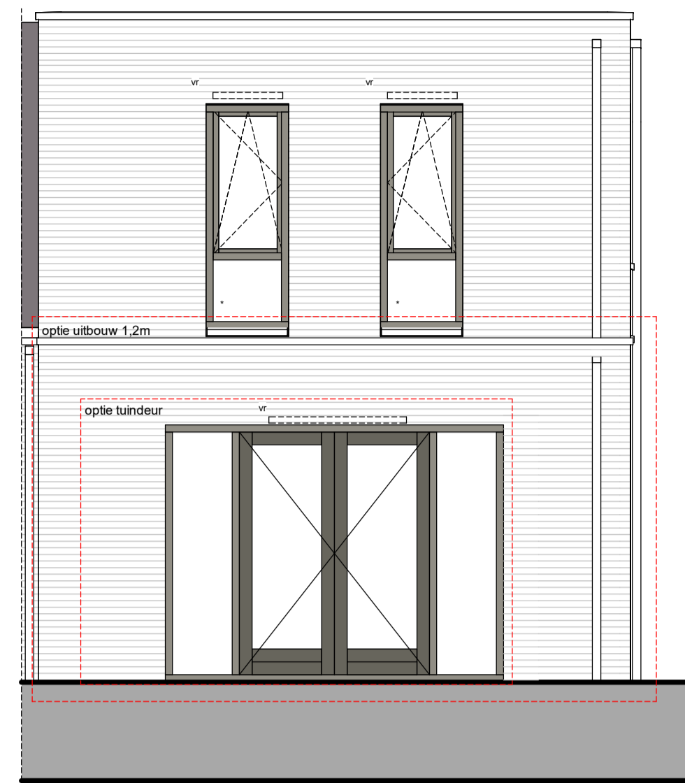
achtergevel
